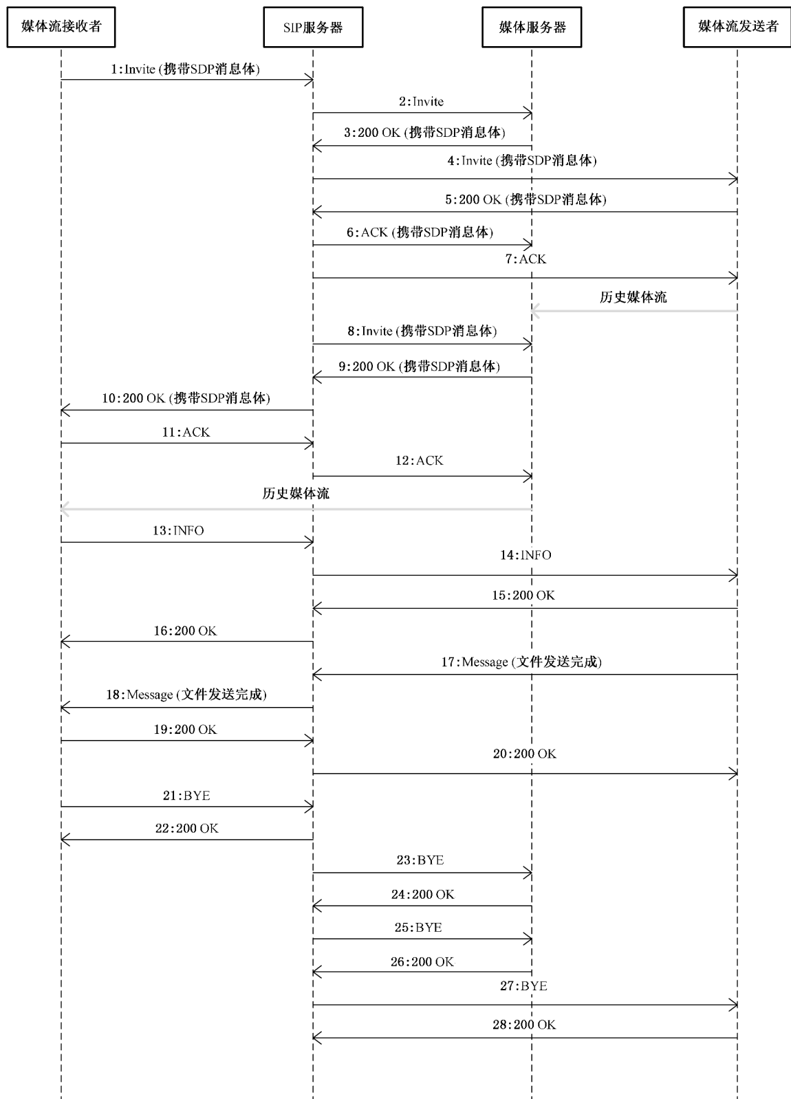
图 19 客户端主动发起的历史音视频回放流程示意图
